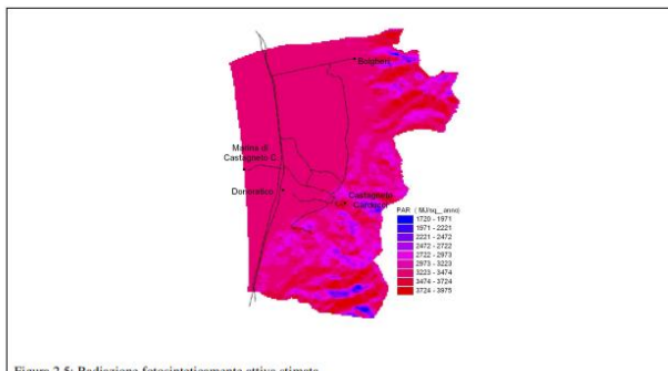
Figura 2.5: Radiazione fotosinteticamente attiva stimata.
