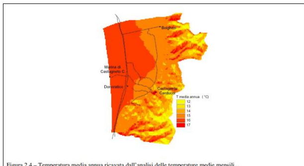
Figura 2.4 – Temperatura media annua ricavata dall'analisi delle temperature medie mensili.
